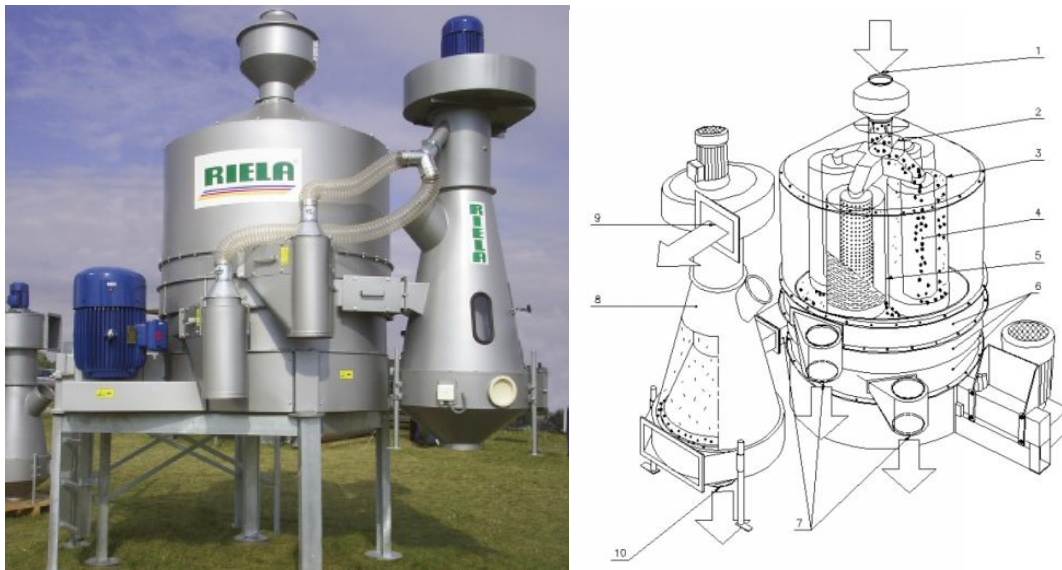
Рис. 3. Роторний сепаратор PROF SEED Німецької фірми RIELA [6]
