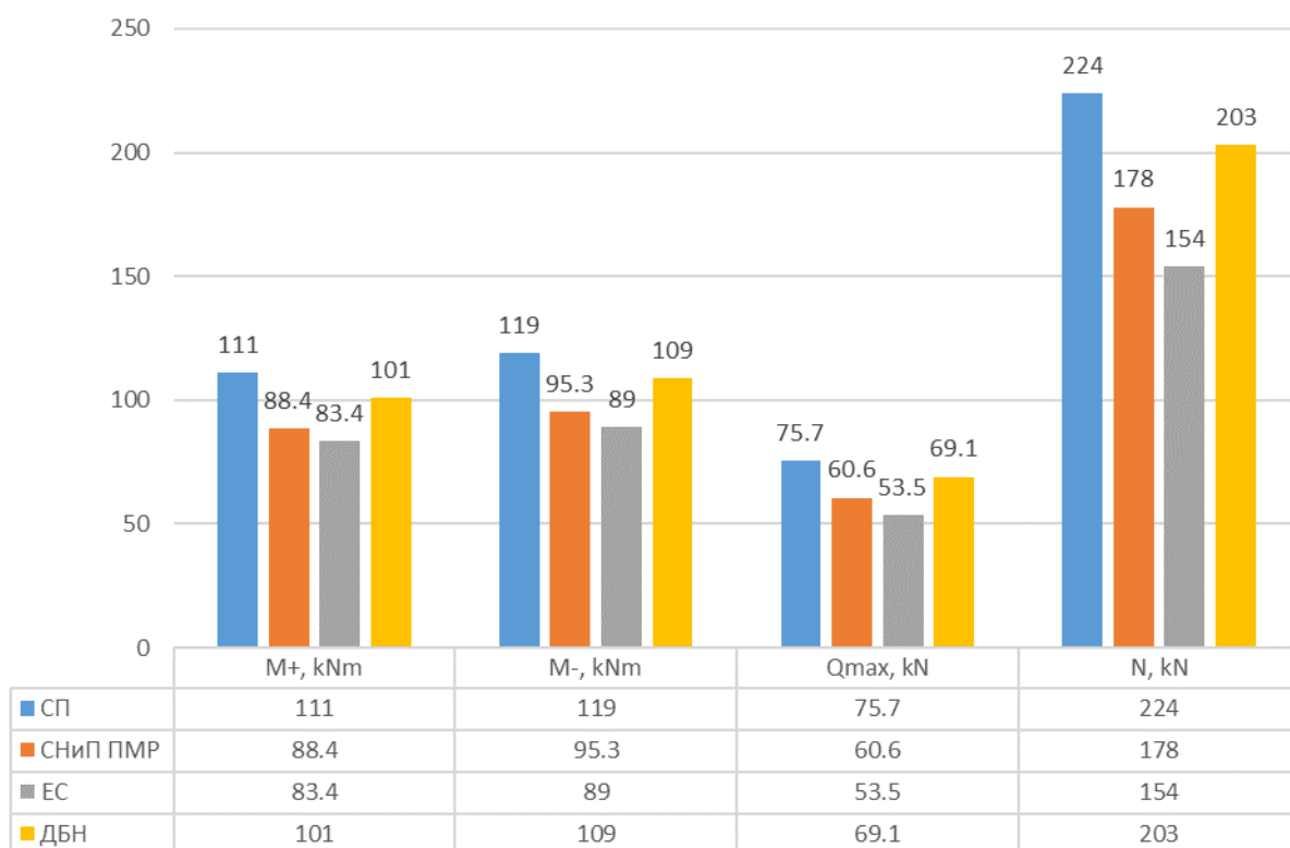
Рис. 2. Максимальные усилия в стержневых элементах схемы для СП 14.13330.2014, СНиП ПМР 22-03-2009, Eurocode 8 и ДБН В.1.1-12:2014
