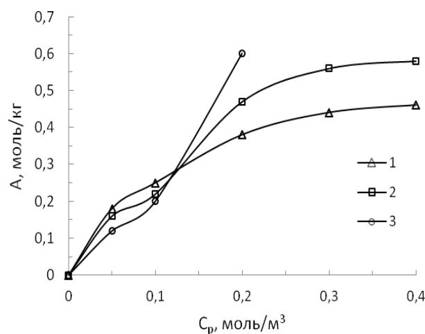
Рис.1. Ізотерми адсорбції ТХ-45 на графітованій сажі при різних температурах, °С: 20 (1); 30 (2) та 45 (3)
