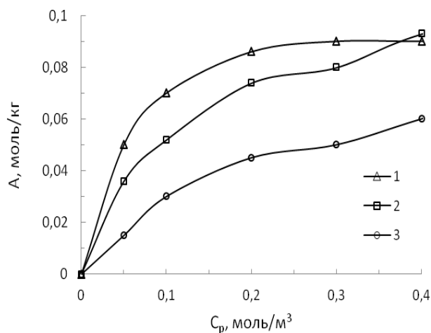
Рис.3. Ізотерми адсорбції TX-305 на графітованій сажі при різних температурах, °С: 20 (1); 30 (2) та 45 (3)
