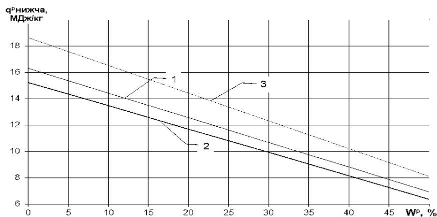
Рис. 6. Залежність нижчої теплоти згоряння двокomпонентних палив на основі соломи від вологості.
