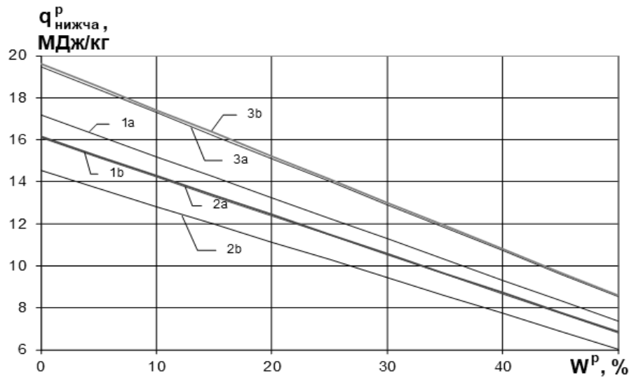
Рис.5. Залежність нижчої теплоти згоряння двокomпонентних палив на основі лушпиння від вологості.
