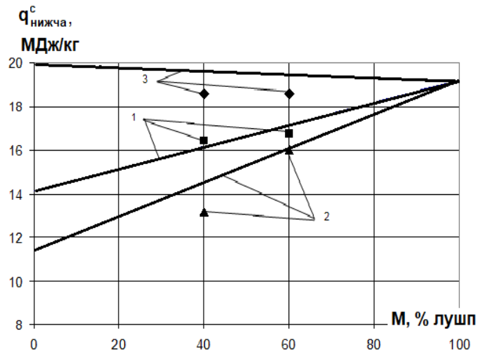
Рис.2. Залежність нижчої теплоти згорання сухих композитних паливних сумішей від вмісту лушпиння соняшнику: 1 – суміш лушпиння і шламу; 2 - суміш лушпиння і курячого посліду; 3 - суміш лушпиння і гною.
