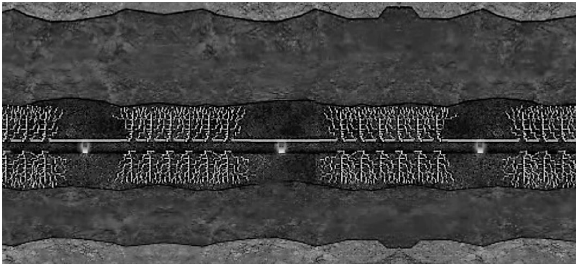
Рис. 1. Схема поінтервального утворення тріщин у пласті при здійсненні гідророзриву в горизонтальній свердловині
